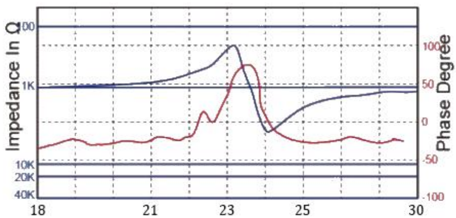
图 2: 阻抗幅度/相位
