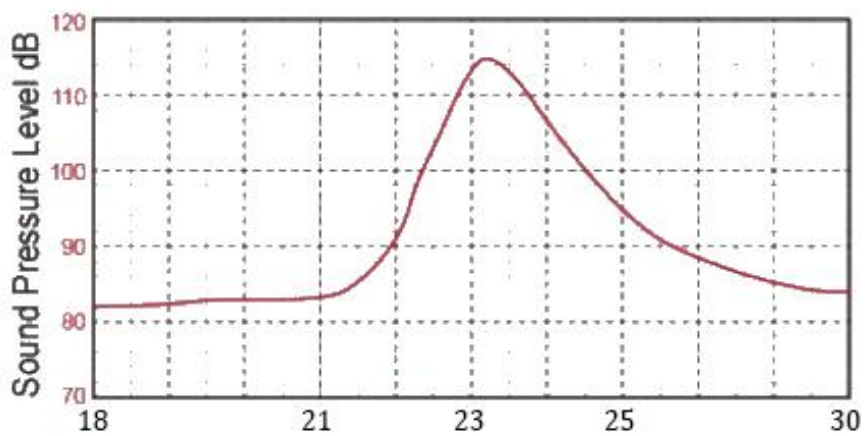
图 3: 声压灵敏度
