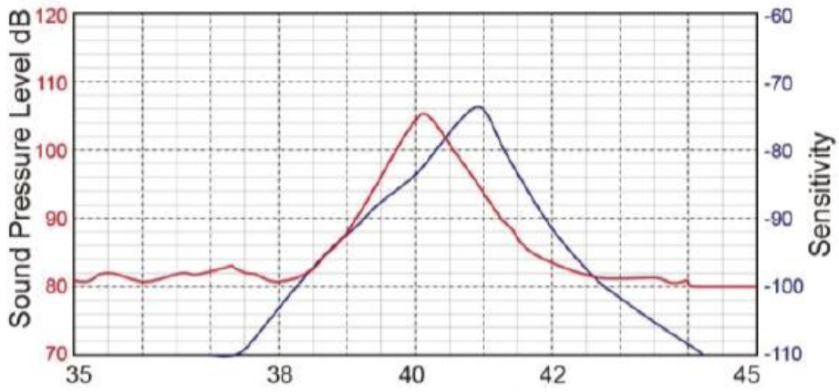
图 3: 声压灵敏度
