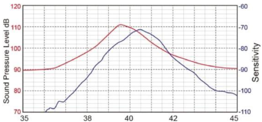
图 3：声压灵敏度
