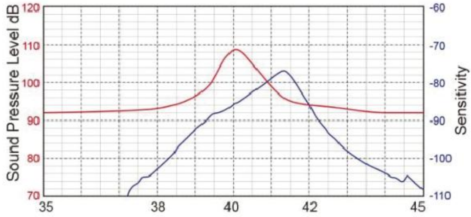
图 3: 声压灵敏度
