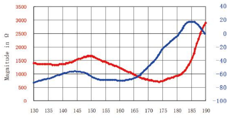
图 2: 阻抗幅度/相位
