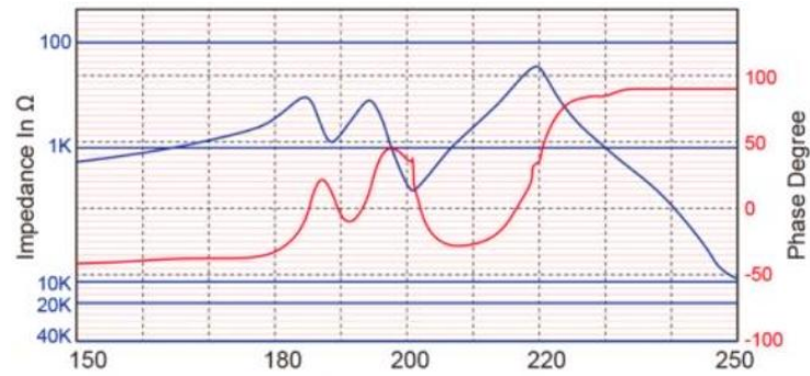
图 2: 阻抗幅度/相位 换个图
