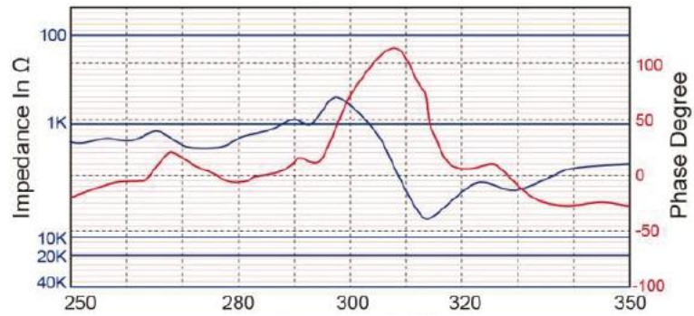
图 2：阻抗幅度/相位
