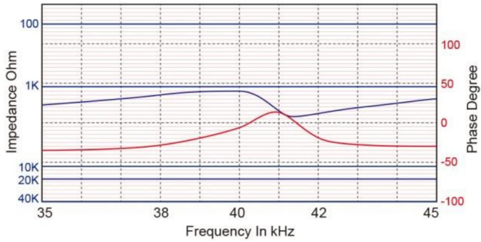
图 2: 阻抗幅度/相位
