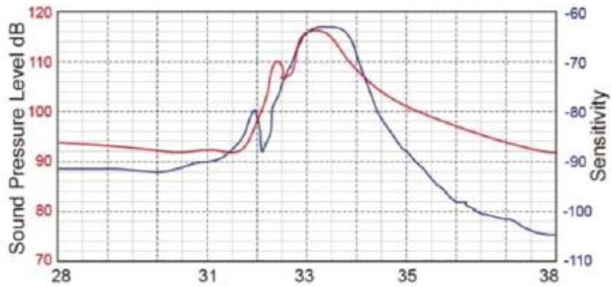
图 3: 声压灵敏度
