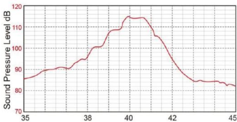
图 3: 声压灵敏度
