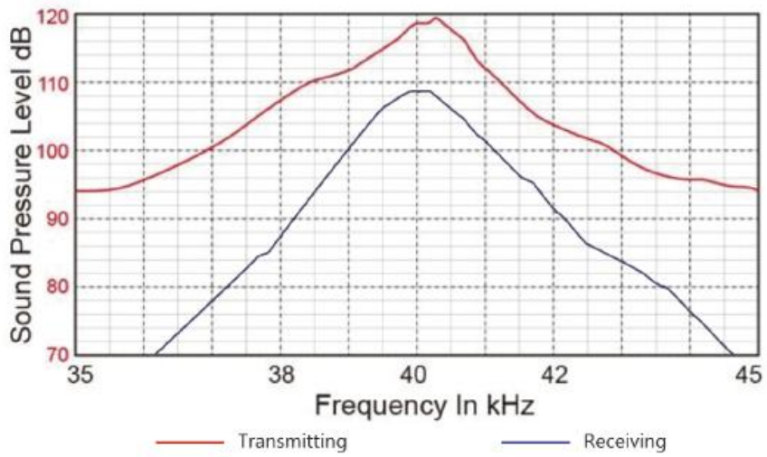
图 3：声压灵敏度
