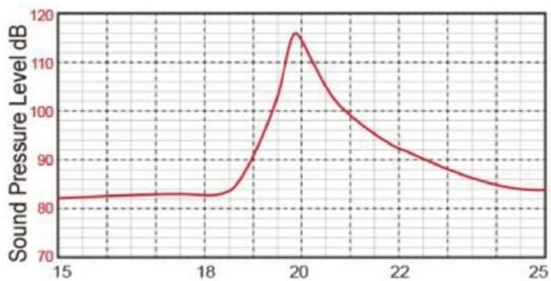
图 3: 声压灵敏度
